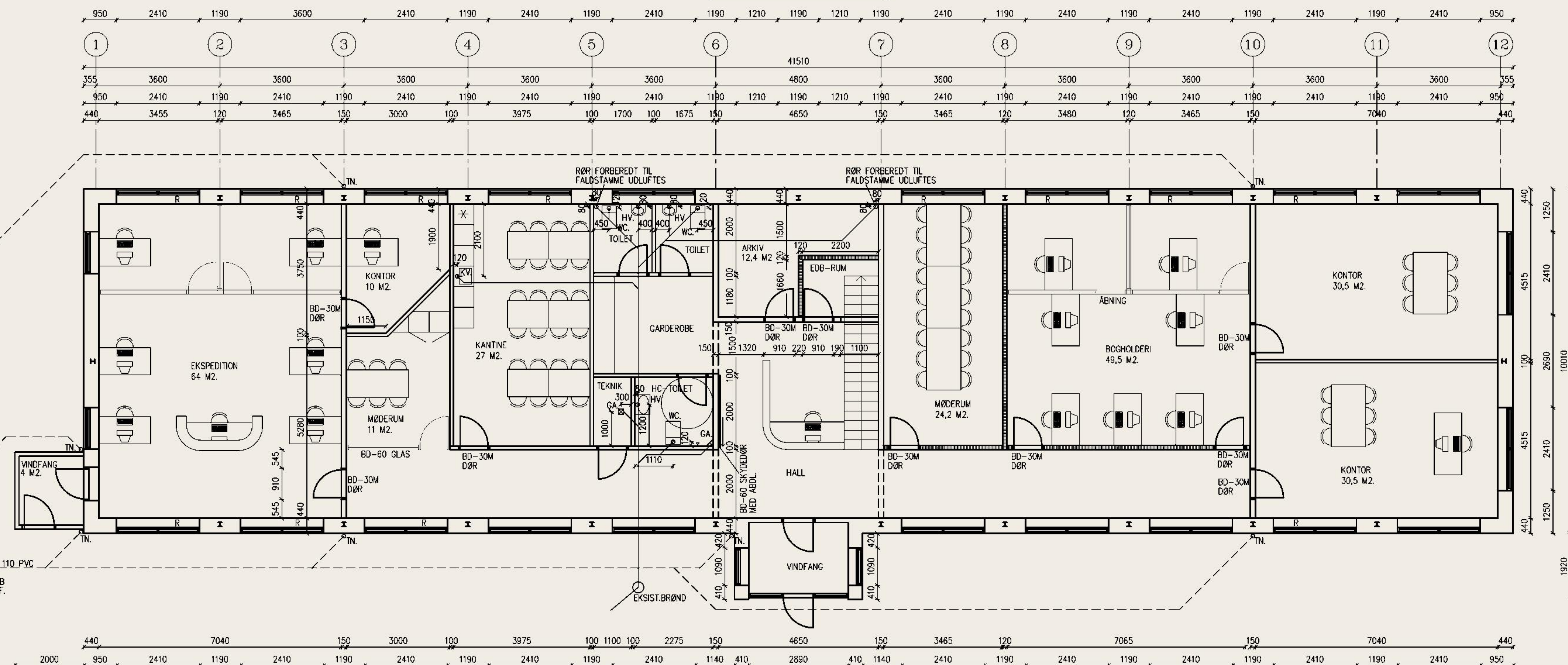
GRUNDPLAN STUEETAGE 422 M2.
