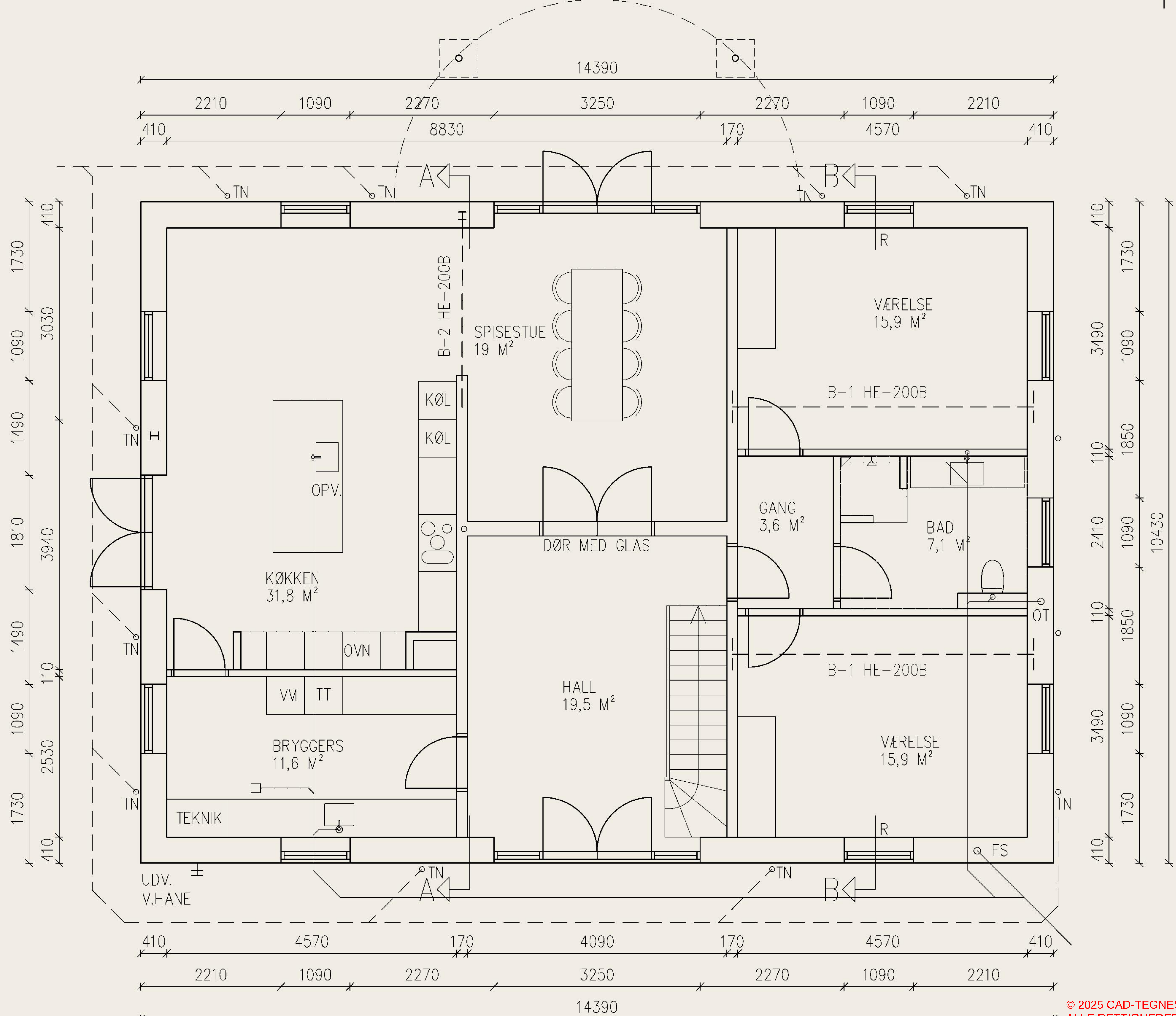
STUEPLAN 150,1 M 2
